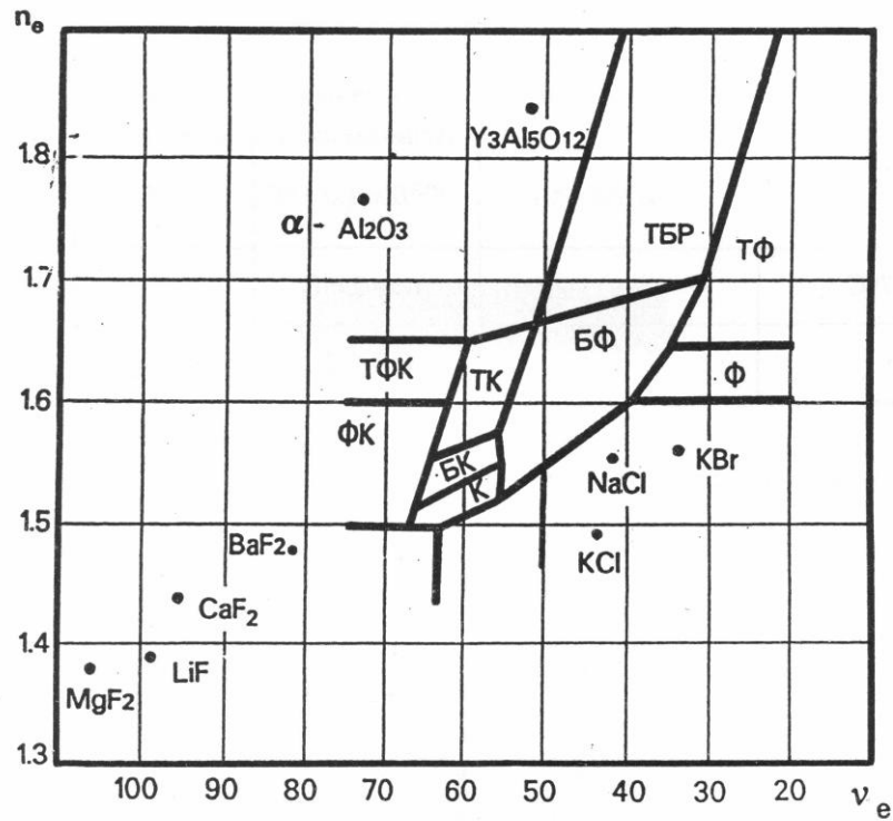
Диаграмма Аббе
