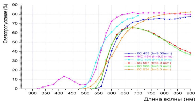
Светопропускание стекол.
